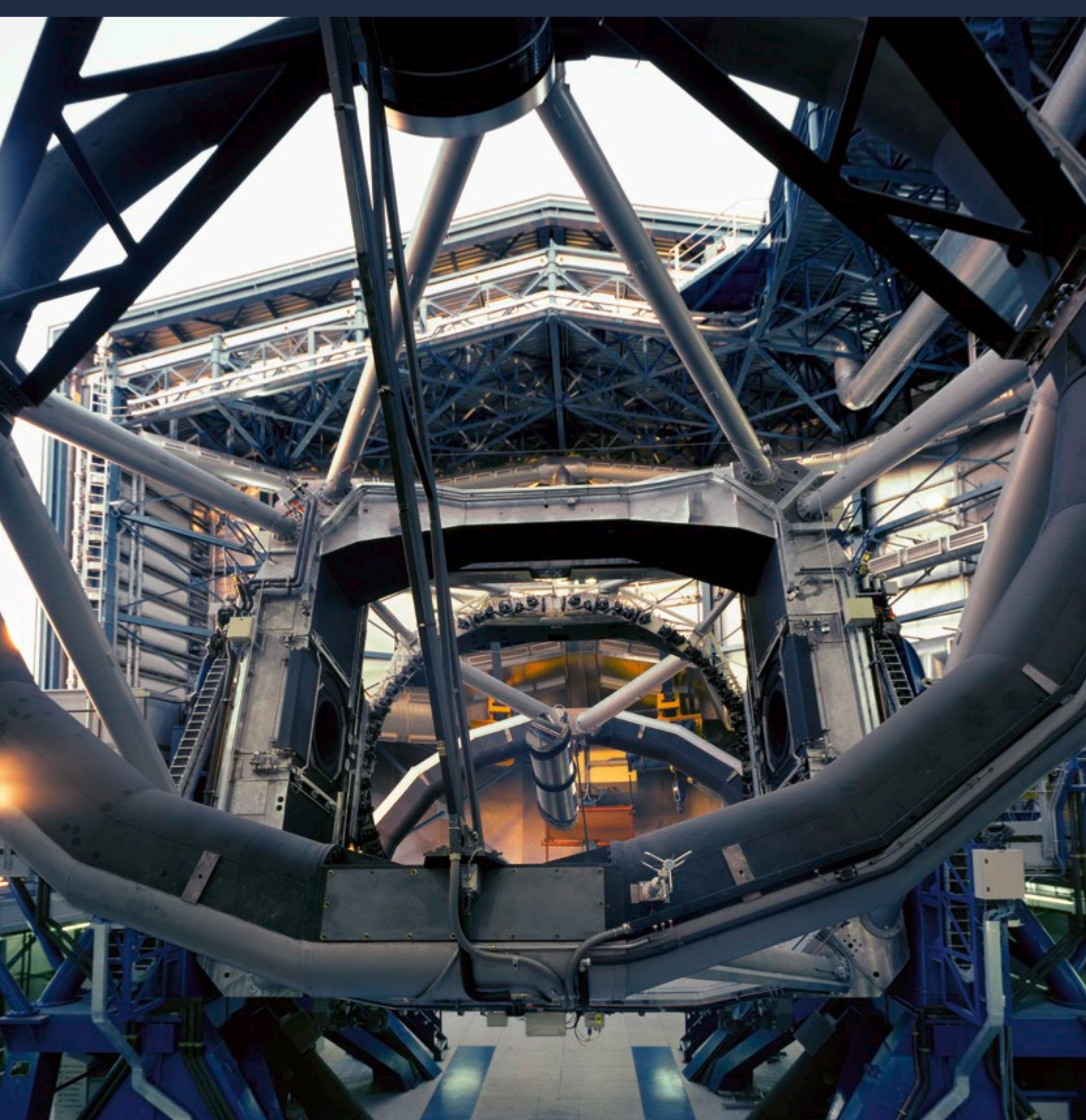
La Unidad de Telescopio 2 del VLT, Kueyen (La Luna). Crédito: ESO/H. H. Heyer
